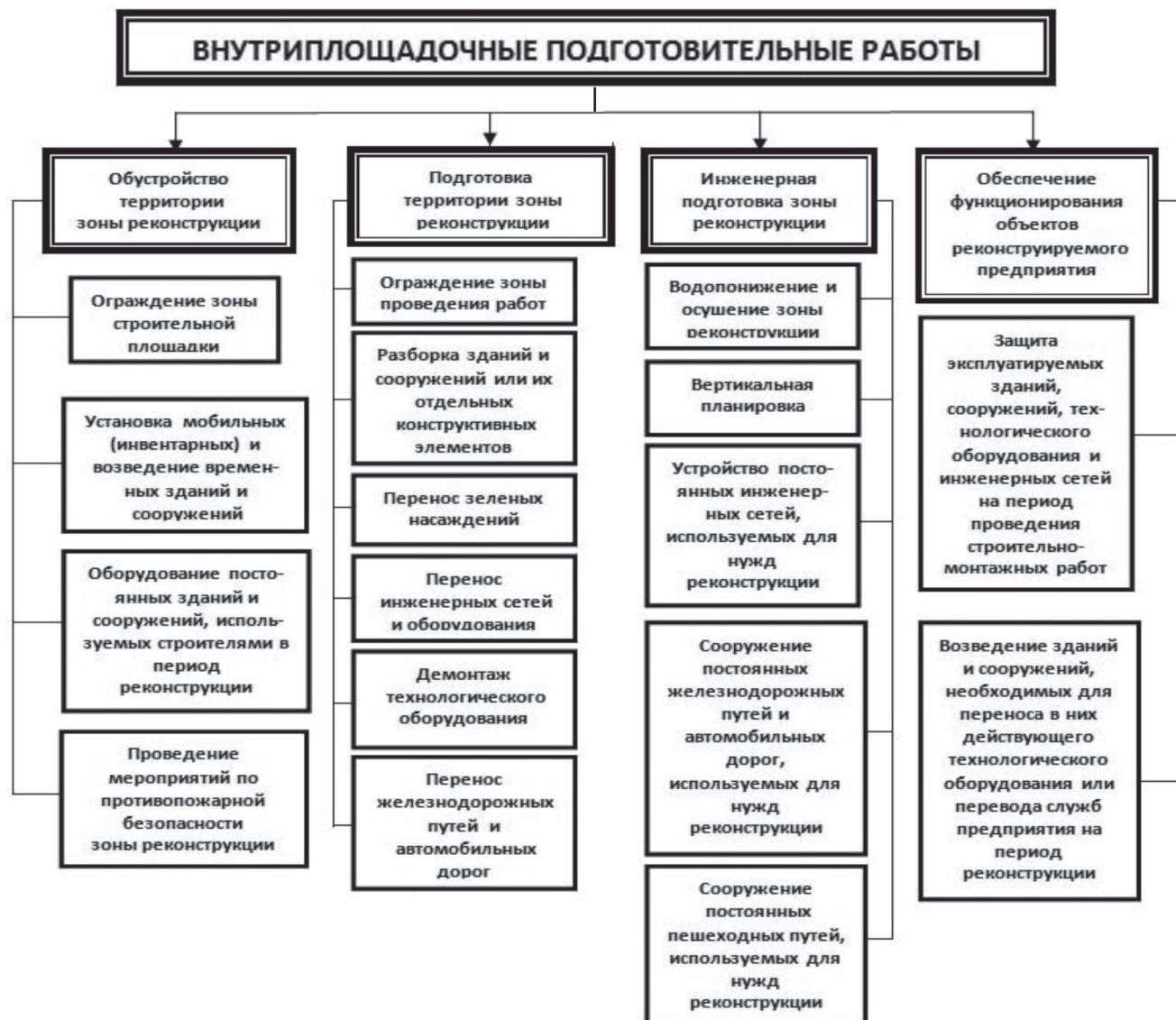
Рисунок 7 – Схема внутриплощадочных подготовительных работ
