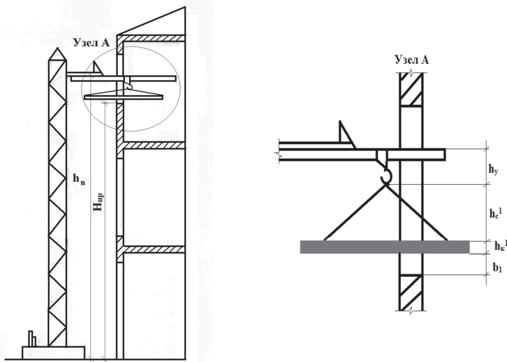
Рисунок 4 – Монтаж конструкций через проемы здания
